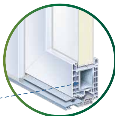
SYSTEM 76 (Ud-Wert 1-tlg. Tür = 1,1 W/m²K)
